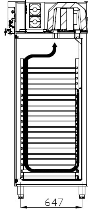
SECTION A-A
