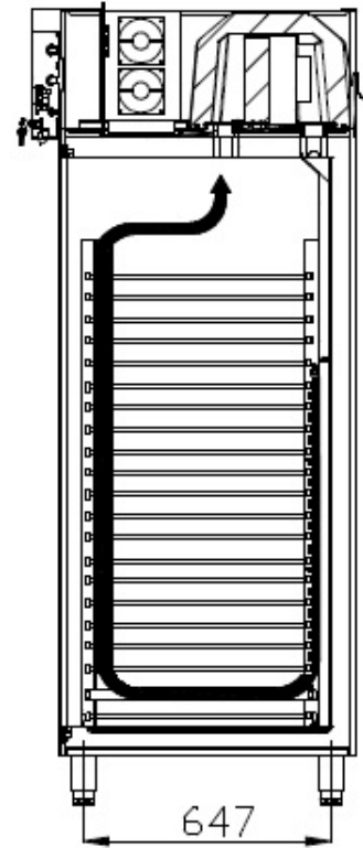
SECTION A-A
