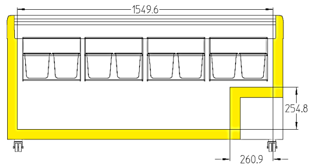
EFI 48.. / EFE51..
