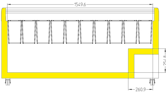
EFI 48.. / EFE51..
