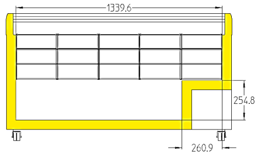
EFI 44.. / EFE 46..
