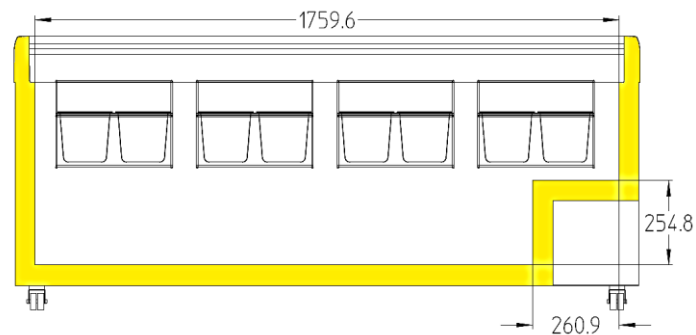
EFI 56.. / EFE60..
