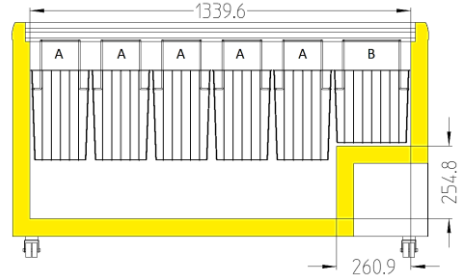
EFE 46..
