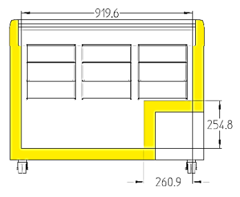
EFI 28.. / EFE 30..
