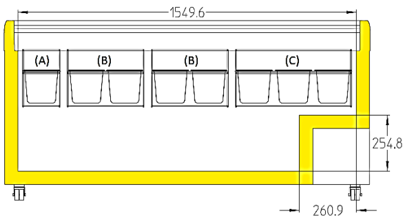
EFI 48.. / EFE51..
