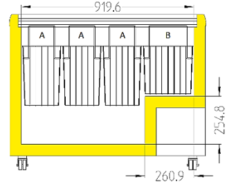
EFE 30..
