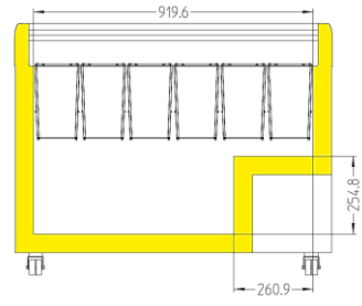
EFI 28.. / EFE 30..
