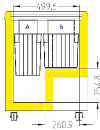
EFE 15..
