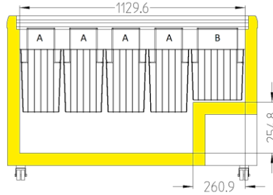
EFE 38..
