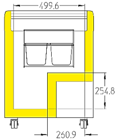
EFI 14.. / EFE15..
