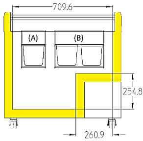
EFI 21.. / EFE22..
