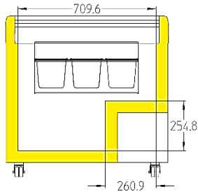
EFI 21.. / EFE22..
