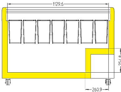
EFI 35.. / EFE38..
