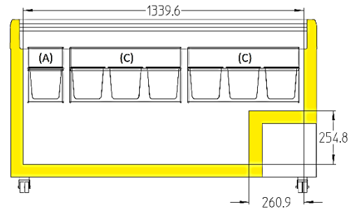
EFI 44.. / EFE 46..
