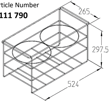
EFI 14.. / EFE15..
