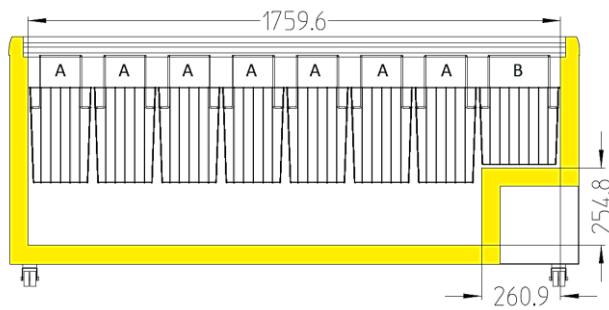
EFE 60..
