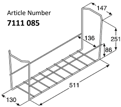
EFI 14.. / EFE15..
