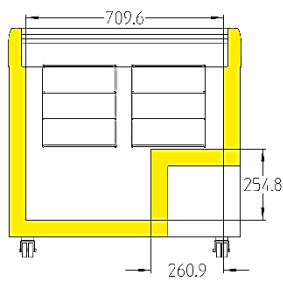
EFI 21.. / EFE22..
