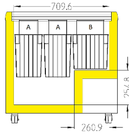
EFE 22..
