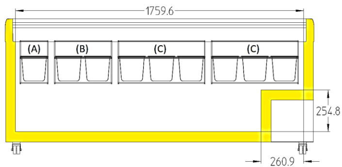
EFI 56.. / EFE60..
