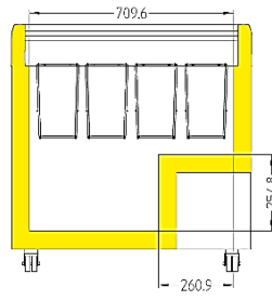
EFI 21.. / EFE22..
