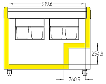
EFI 28.. / EFE 30..
