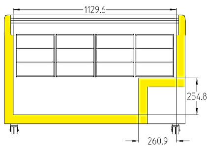
EFI 35.. / EFE 38..
