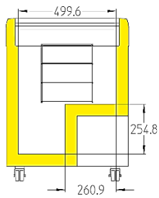
EFI 14.. / EFE15..
